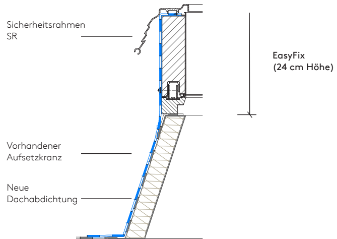
Aufstocksystem EasyFix im Schnitt
