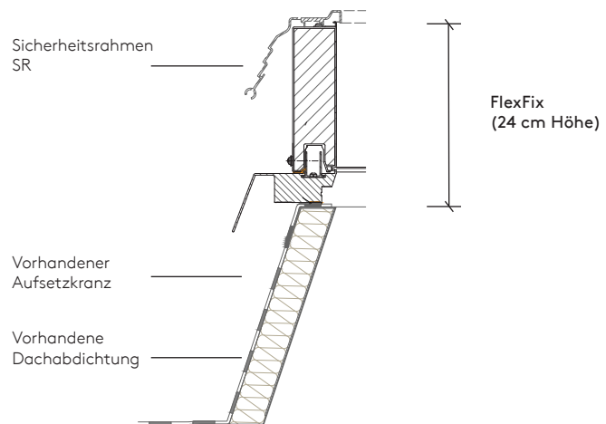
Aufstocksystem FlexFix im Schnitt
