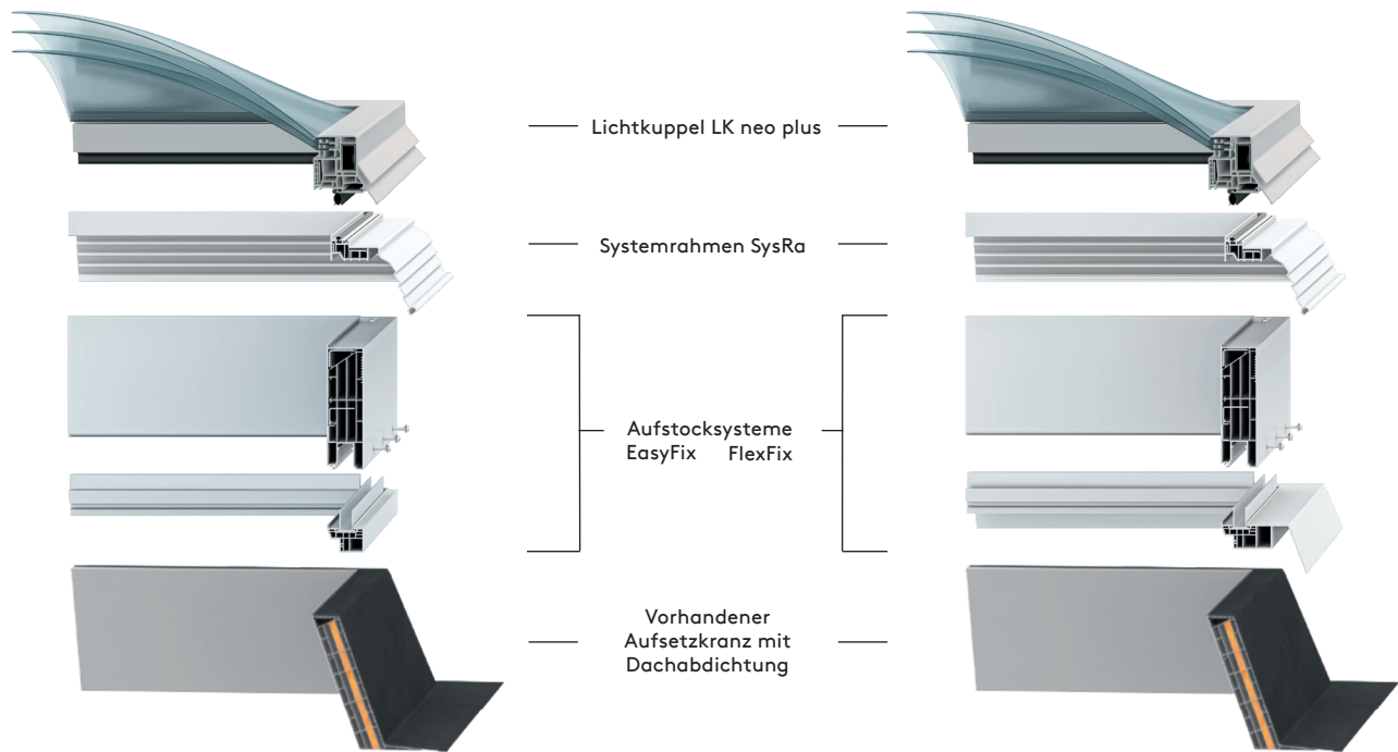
Aufstocksystem EasyFix, 24 cm Höhe Aufstocker und Montagerahmen
