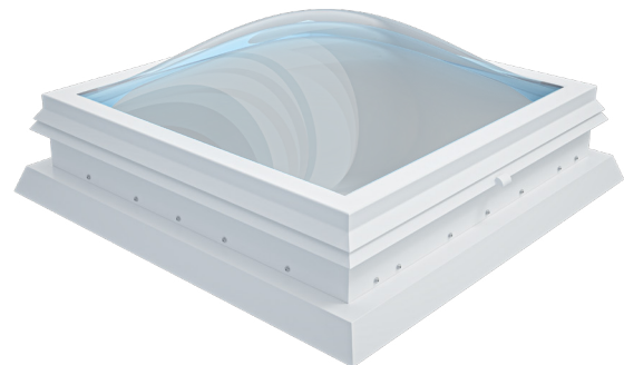
Aufstocksystem FlexFix mit Wetterschutzkante, Systemrahmen SysRa und Lichtkuppel LK neo plus
